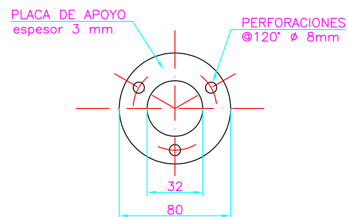
DETALLE PLACA DE APOYO
