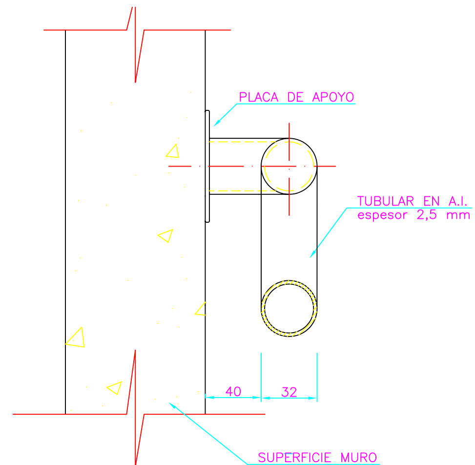
CORTE A-A BARRA ANGULO 120
