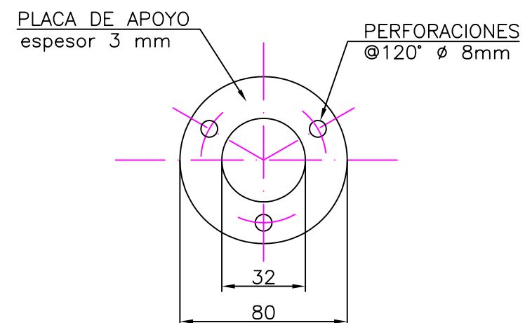
DETALLE PLACA DE APOYO
