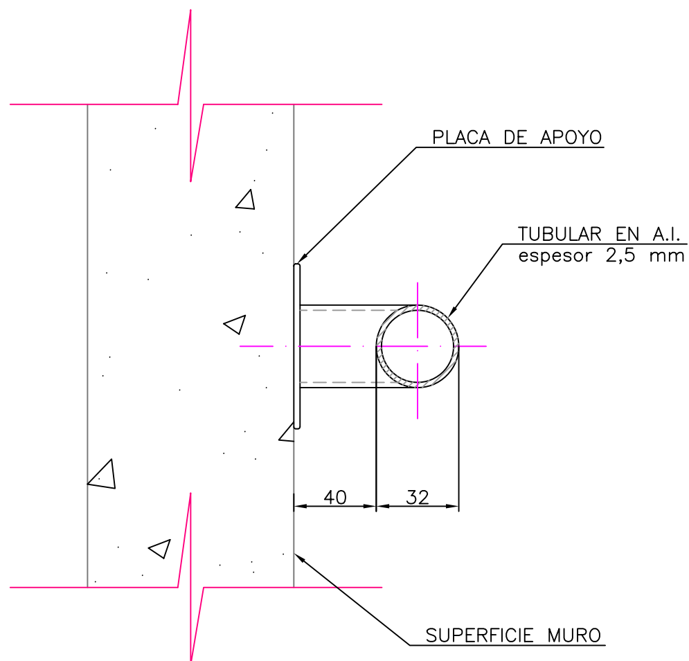
CORTE A-A BARRA RECTA
